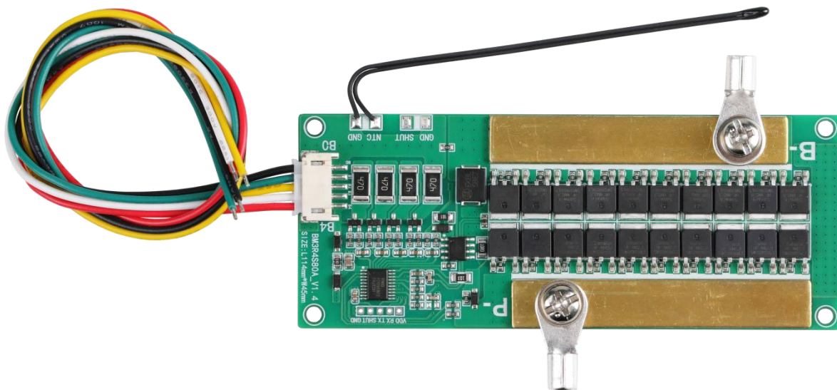
正面图
